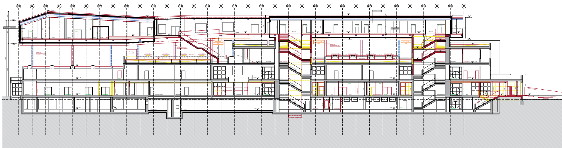
Schnitt
